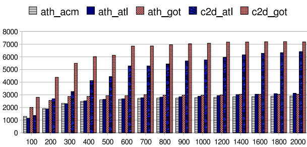
(d) DPOTRF (Cholesky), NB=64
